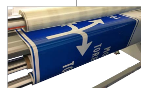
Albero riavvolgitore posteriore con frizione e barra di stacco (optional)
